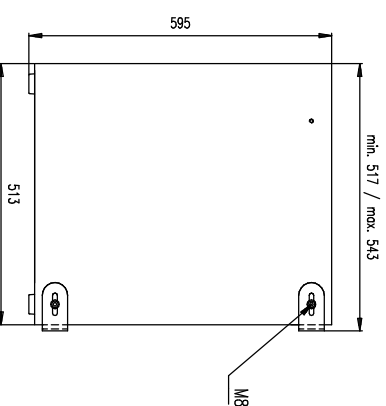
Rückansicht / Rear view Variante 3 / Variation 3
