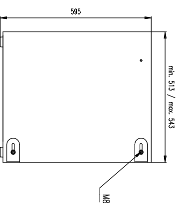
Rückansicht / Rear view Variante 4 / Variation 4
