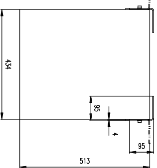
Draufsicht V. 3 u. 4 / Top view V. 3 u. 4
