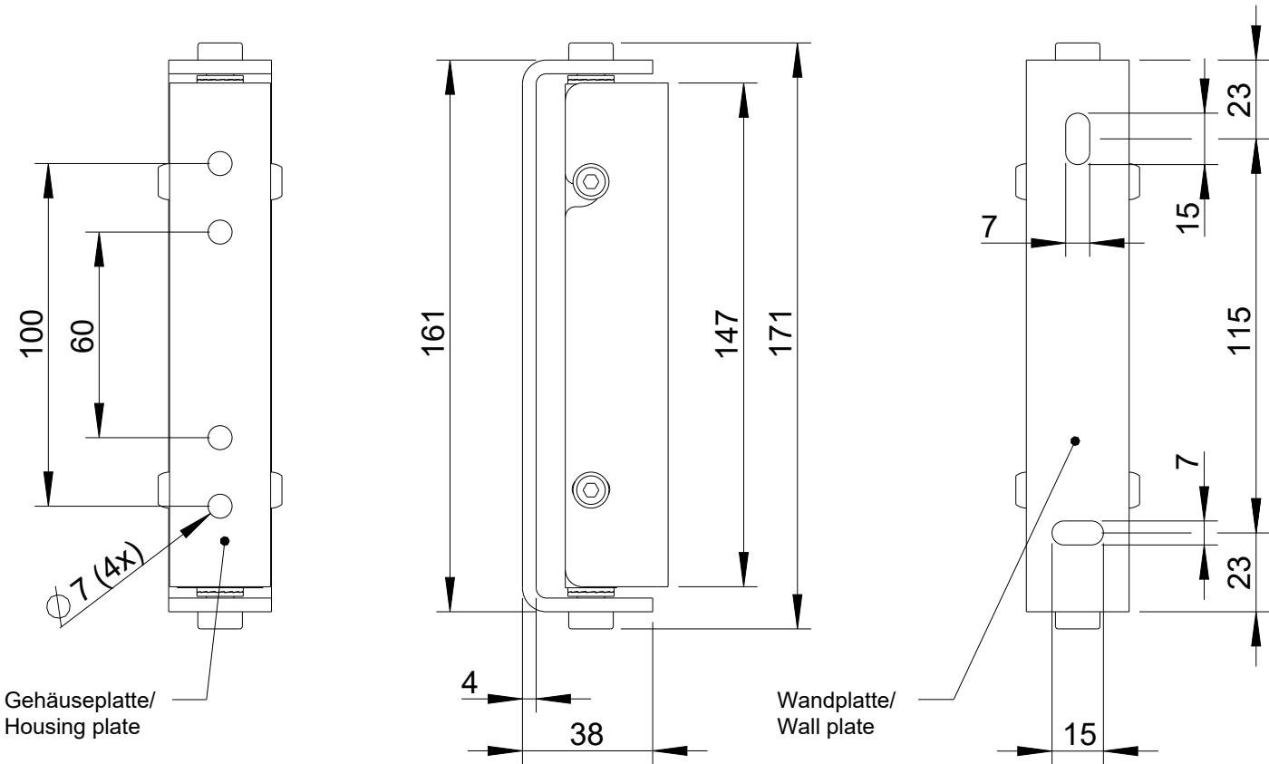
Vorderansicht/ Front view
