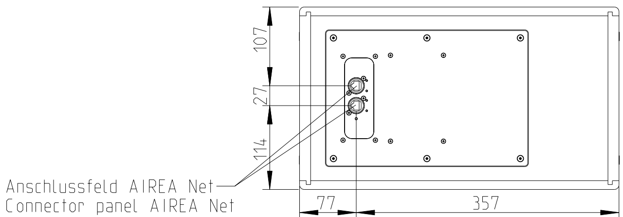
Rückansicht / Rear view
