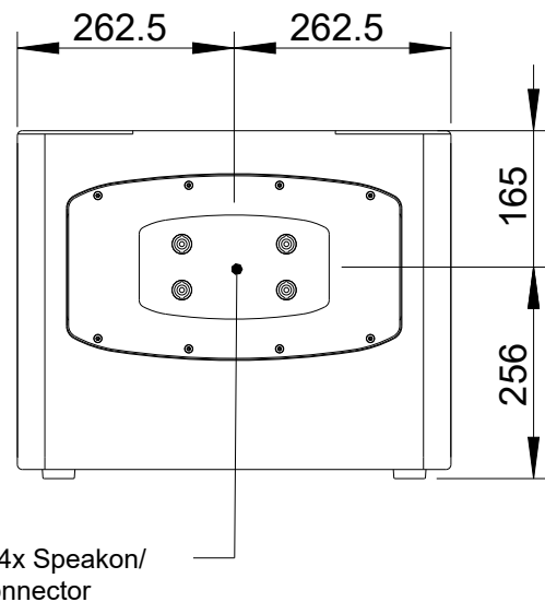
Rückansicht/ Rear view
