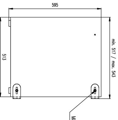
Rückansicht / Rear view Variante 3 / Variation 3
