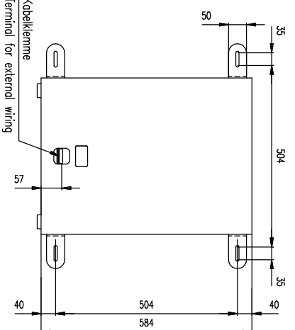
Rückansicht / Rear view Variante 4 / Variation 4
