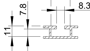
T-Nut/ T-slot
