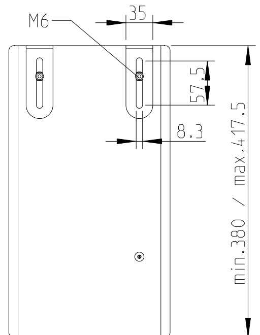
Seitenansicht / Side view
