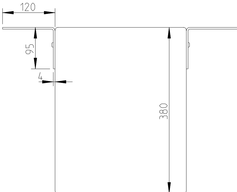
Draufsicht / Top view
