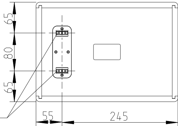
Rückansicht / Rear view
