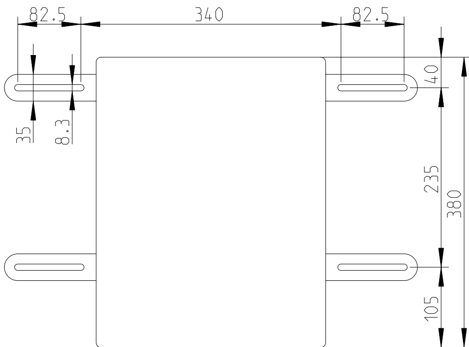
Draufsicht / Top view
