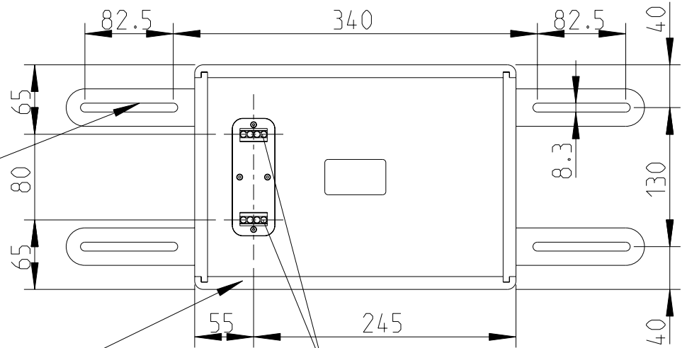
Rückansicht / Rear view
