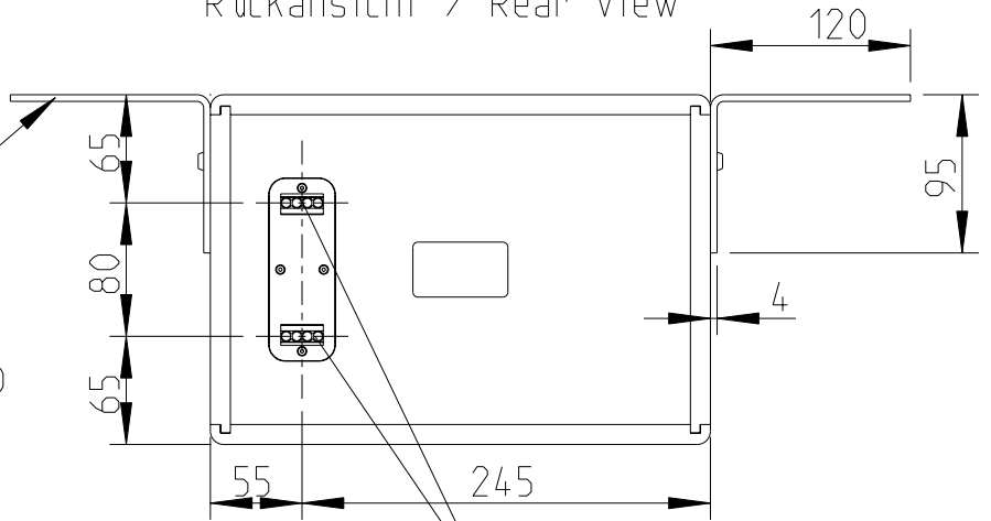
Rückansicht / Rear view
