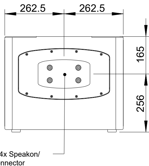
Rückansicht/ Rear view
