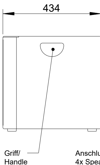
Seitenansicht/ Side view
