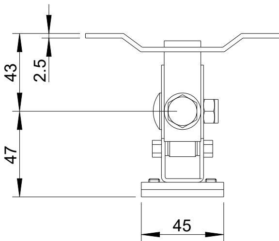
Draufsicht / Top view
